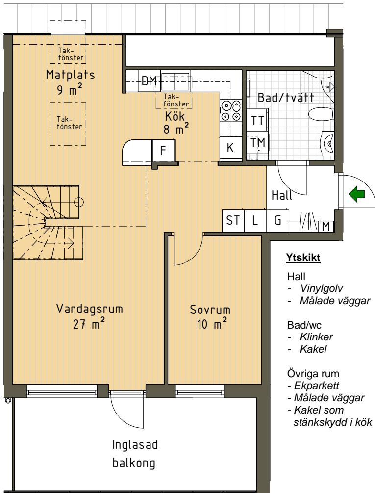
Våning 5
